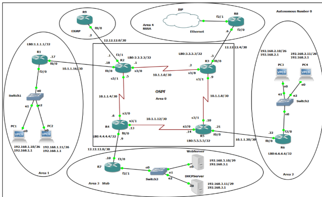
Fig. 5. OSPF scenario in GNS3
